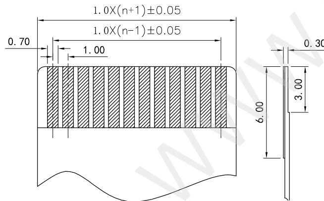
适用FFC寸法 Applicable FFC
