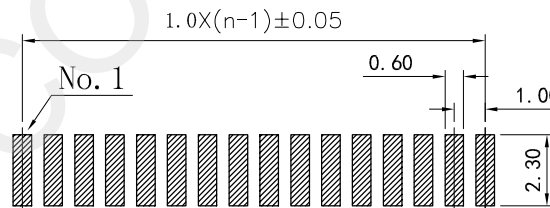
PCB 寸法 PCB Layout
